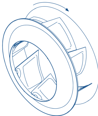
Drehrichtung / Direction of rotation Bsp: saugseitig gesehen: Rechtslauf (R)/ example: suction side view: clockwise rotation (R)
